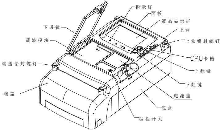
图 2：外形布局图
