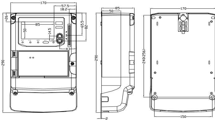
图 3：安装尺寸图
