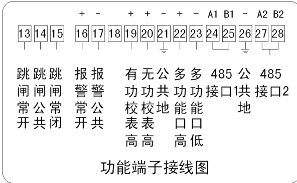
图 7 电能表辅助端子排列图
