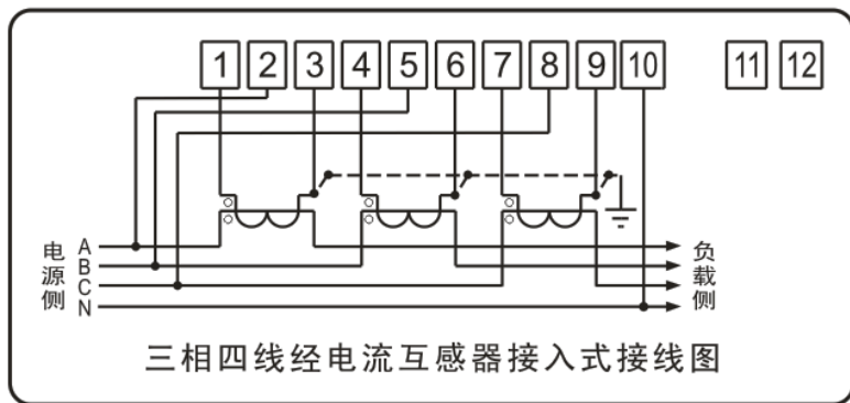
图 4：接线图
