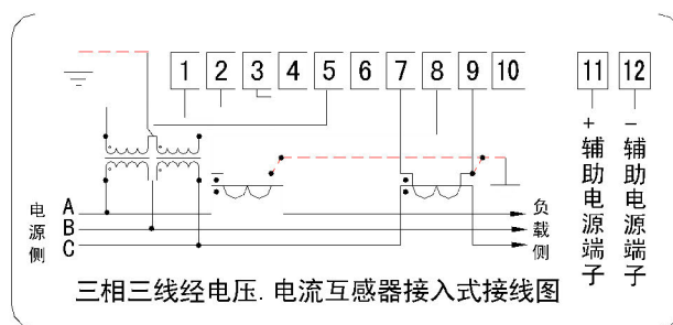
图 4：接线图
