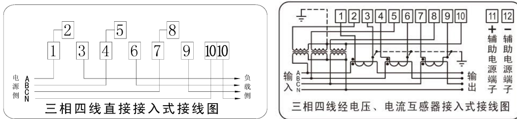
图 2：主端子接线图
