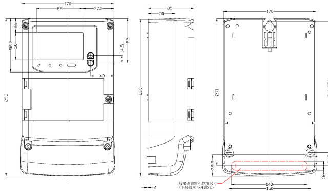
图 1：安装尺寸图
